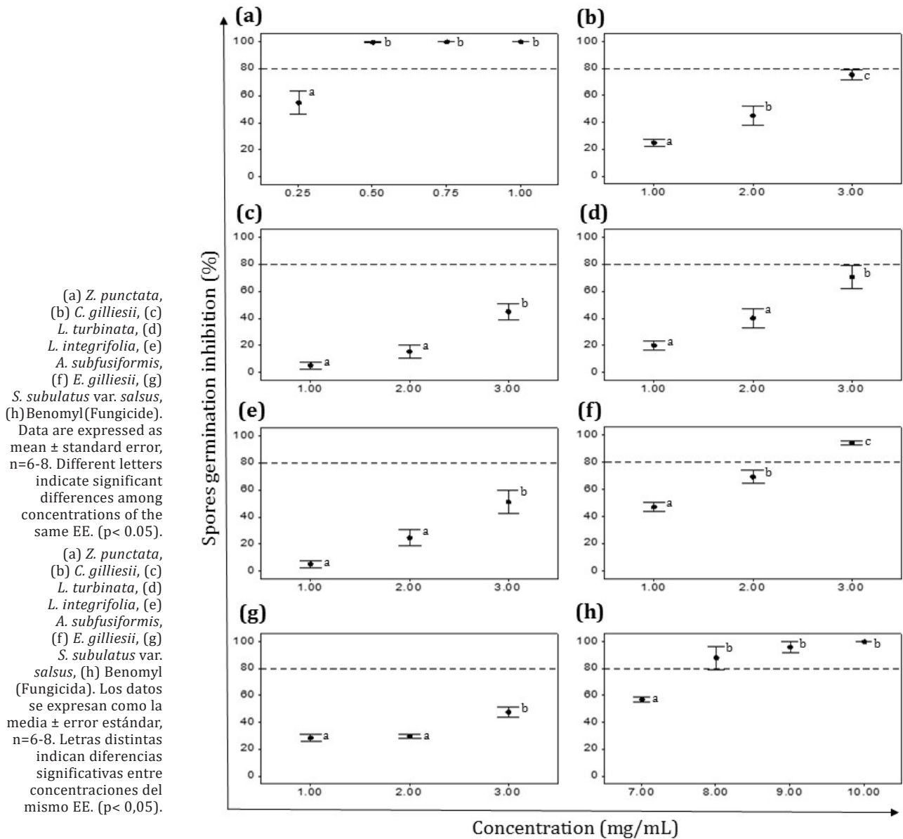
Figure 3. Effect of ethanolic extracts (EEs) on P. parasiticum spore germination. Figura 3. Efecto de los extractos etanólicos (EEs) sobre la germinación de esporas de P. parasiticum .
